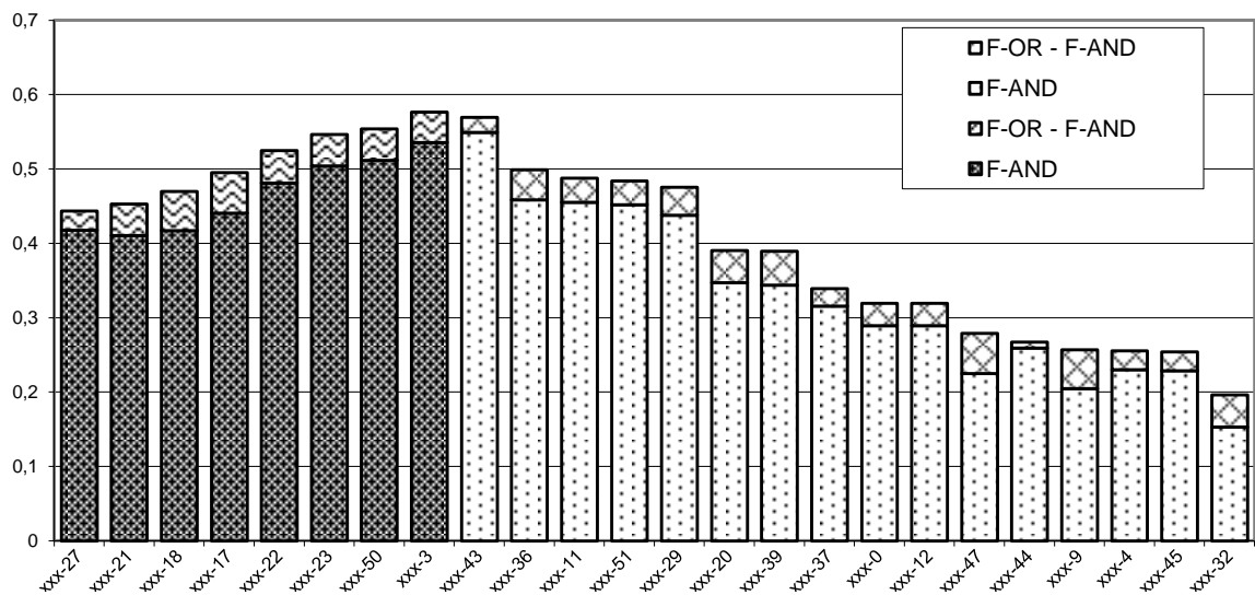
Рис. 3. Результаты оценки прогонов дорожки классификации на 3 класса.
