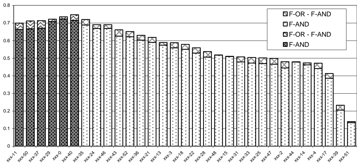
Рис. 2. Результаты оценки прогонов дорожки классификации на 2 класса.
