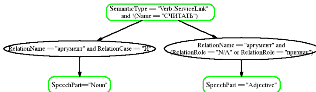
Рис. 1. Пример семантического шаблона для определения оценки книги.
